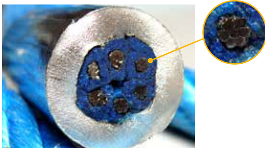
Intérieur de la corde avec 6 coeurs d'acier 6/36.
